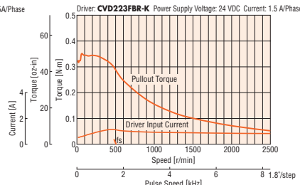
PKP243D15A2/ PKP243D15B2
