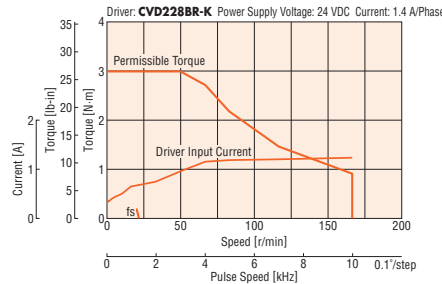
PKP264D14A2-SG18/PKP264D14B2-SG18
