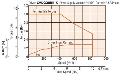
PKP264D28A2-SG10/ PKP264D28B2-SG10
