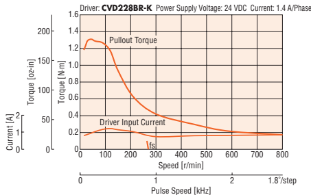
PKP266D14A2/PKP266D14B2
