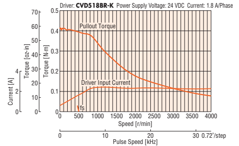
PKP545N18A2-R2GL/ PKP545N18A2-R2G
