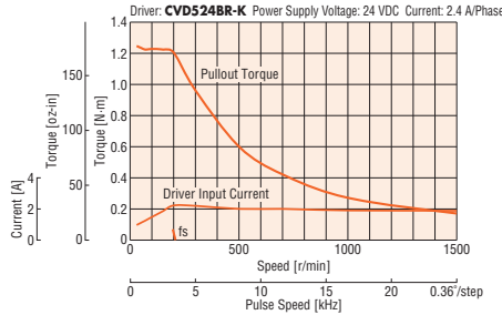
PKP566FMN24A/PKP566FMN24B
