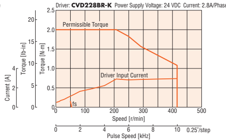
PKP264D28A2-SG18/ PKP264D28B2-SG18
