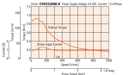
PKP246D15A2/ PKP246D15B2
