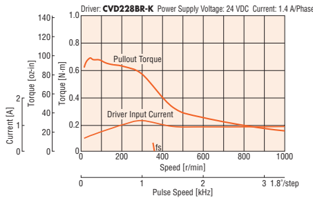
PKP264D14A2/PKP264D14B2
