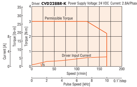
PKP264D28A2-SG18/ PKP264D28B2-SG18
