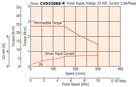
PKP264D28A2-SG10/ PKP264D28B2-SG10
