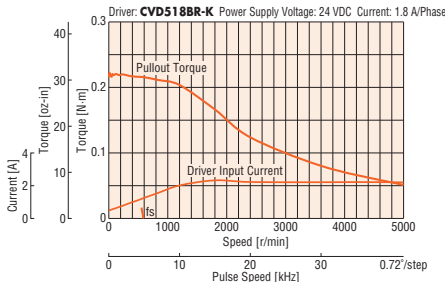
PKP546N18A2/ PKP546N18B2
